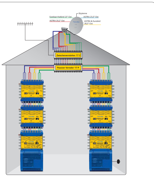
Installationsbeispiel
